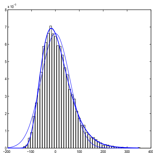
Obrázek 1: Hustota statistiky \sqrt{n}(\bar{e}^{\bar{X}_n} - e^\mu) : skutečná (tučná čára), asymptotická (slabá čára) a bootstrapová (histogram).
